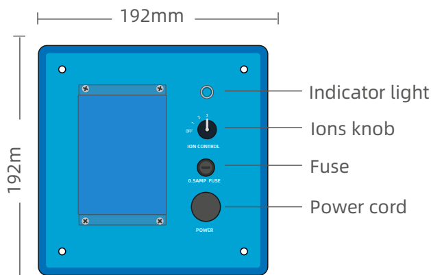
Ion generator
